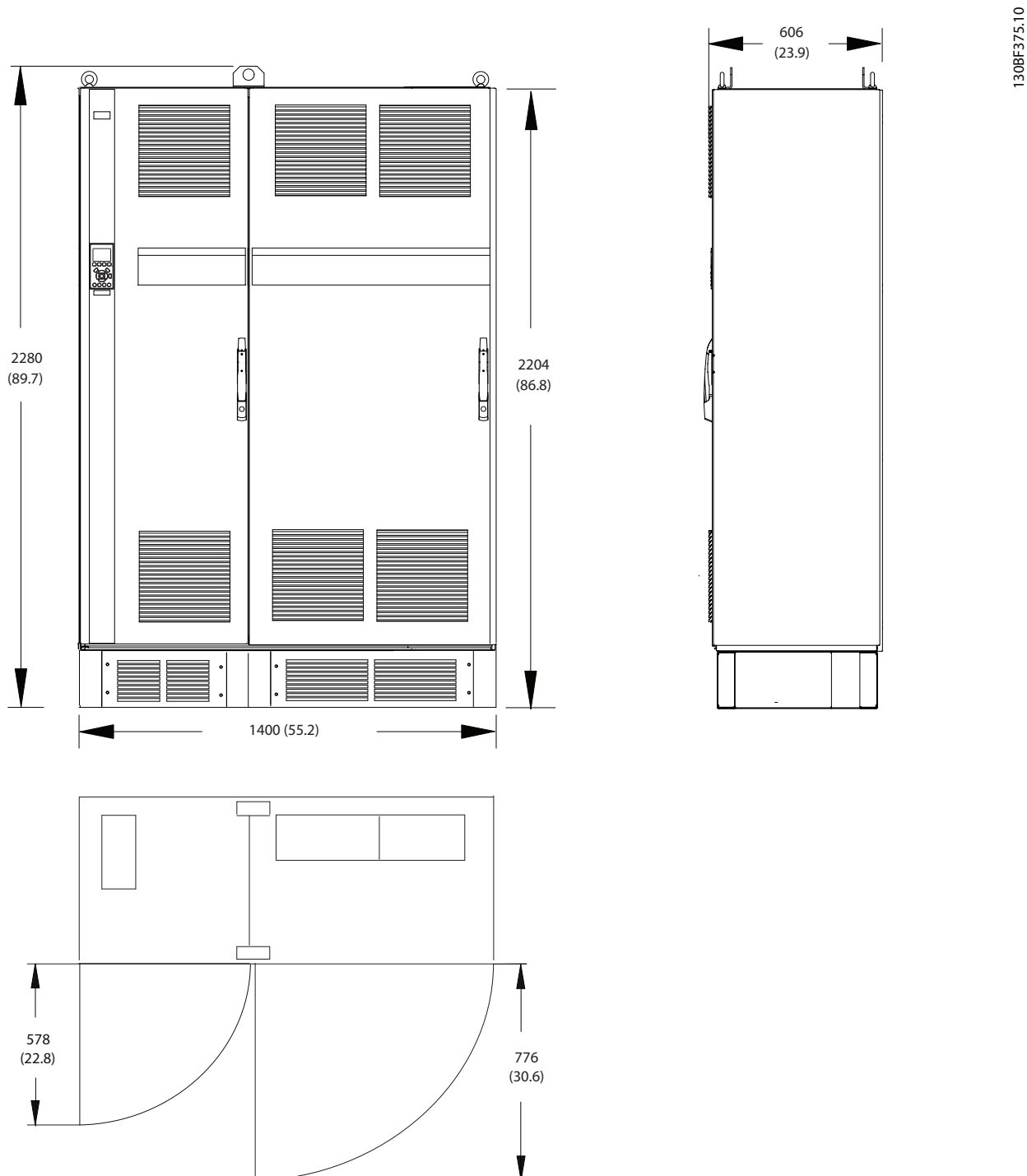
Ilustração 8.19 Dimensões da folga da porta, frontal e lateral do F1
