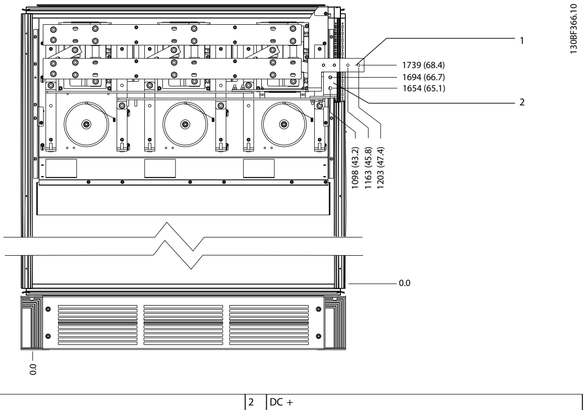
Ilustração 8.32 Dimensões do terminal para os terminais de regeneração F2/F4, vista frontal
