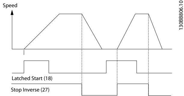
Ilustração 8.3 Partida por pulso/Parada por inércia inversa
