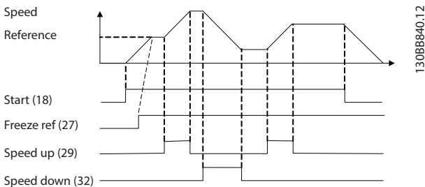
Ilustração 8.4 Aceleração/desaceleração
