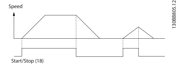
Ilustração 8.2 Partida/parada com Safe Torque Off
