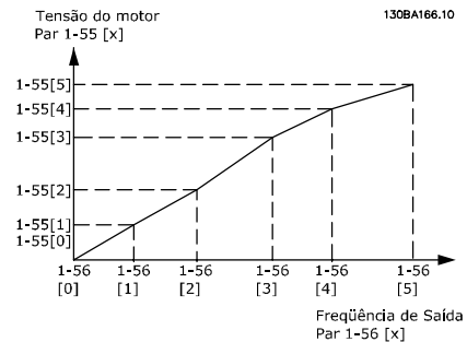
Ilustração 4.1 Características U/f
