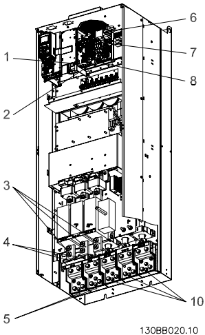
Ilustração 3.45: IP 00 Compacto (Chassi) com desconexão, fusível e filtro de RFI, tamanho de chassi E2
