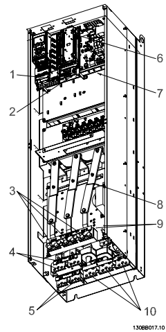
Ilustração 3.40: IP 00 Compacto (Chassi), tamanho de chassi D3
