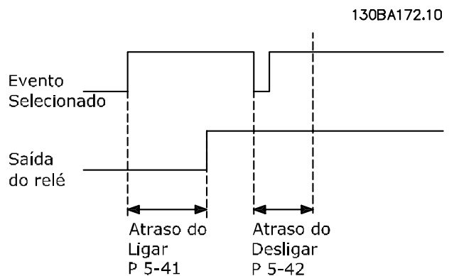
Ilustração 3.8 Atraso de desativação do relé
