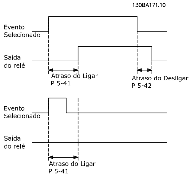
Ilustração 3.7 Atraso de ativação do relé
