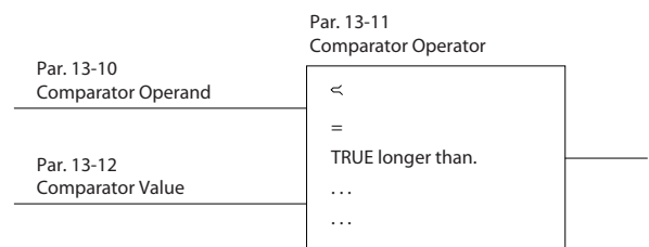
Ilustração 3.14 Comparadores
